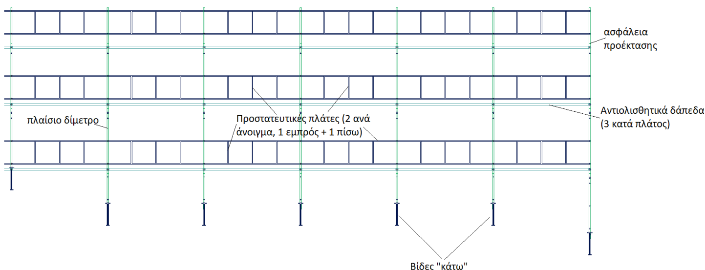
Εικόνα 12: Σκαρίφημα όψης με την τελική εικόνα των ικριωμάτων όπως αυτά θα τοποθετηθούν από εργαζομένους της Εφορείας Αρχαιοτήτων Λέσβου κατά την διάρκεια του έργου.
