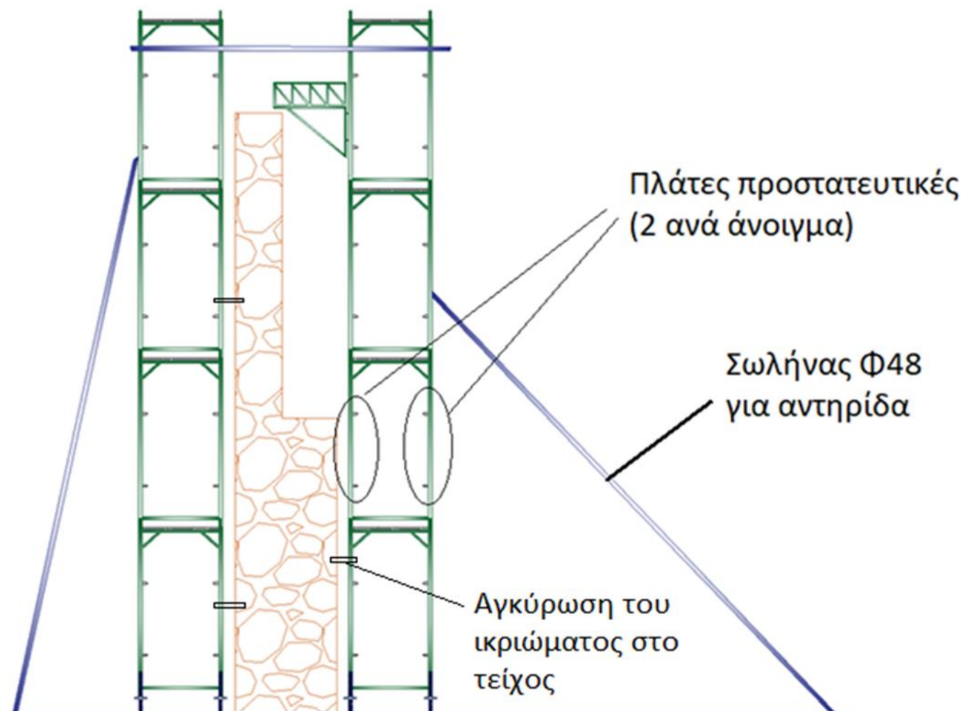
Εικόνα 1: Σκαρίφημα με ενδεικτικό τρόπο τοποθέτησης ικριωμάτων στο επιθαλάσσιο τείχος του Κάστρου Μυτιλήνης.
