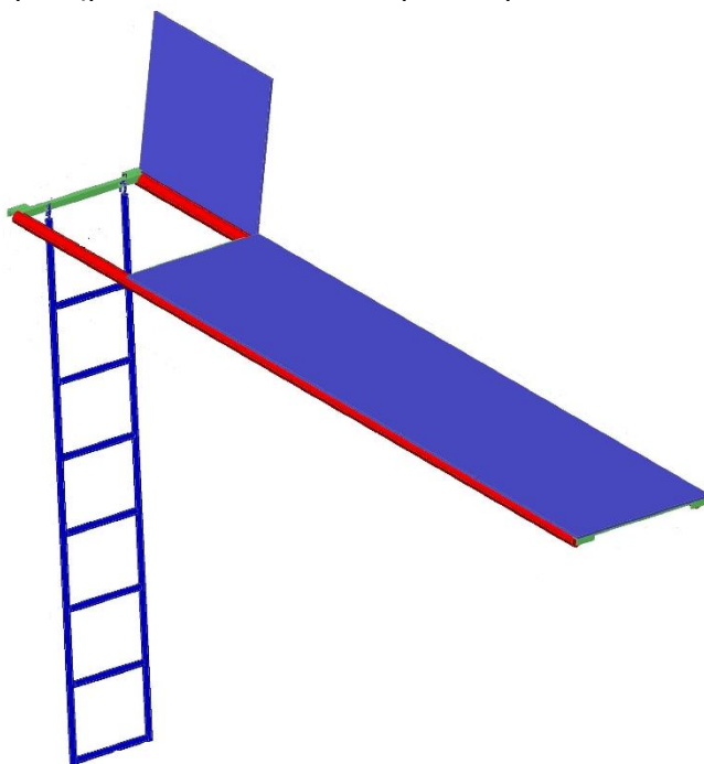
Εικόνα 8: Πλατφόρμα εργασίας με καταπακτή και ενσωματωμένη σκάλα.
